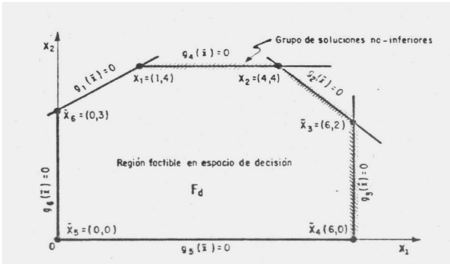
Figura 3. Región factible y soluciones no-inferiores en el espacio de decisión F_d
