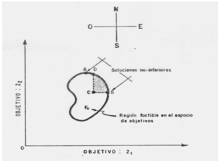
Figura 2. Ejemplo gráfico de soluciones no-inferiores.
