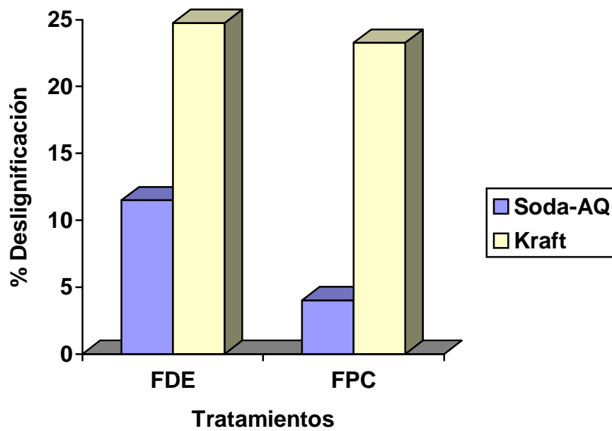
Figura 2. Comparación del porcentaje de deslignificación entre pulpas Soda-AQ y Kraft utilizando cepas de hongos de la pudrición blanca para 15 días de incubación.* Los datos de la pulpa Kraft fueron tomados de Cervantes, R. 1993.
