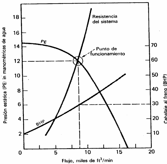
Fig. 1. Punto real de funcionamiento de un ventilador
