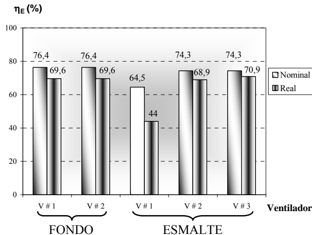
Fig. 5. Comparación de la eficiencia estática nominal y real de los ventiladores centrífugos
