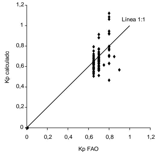
Figura 6. Relación entre K_p tabulado y K_p calculado durante el período 2 (julio-noviembre 2001).
