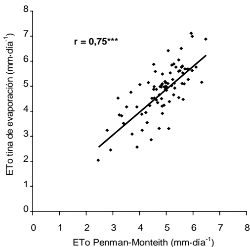
Figura 1. Valores diarios de ET_0 usando los métodos de Penman-Monteith y tina de evaporación en el período 1 (abril-julio 2001).
