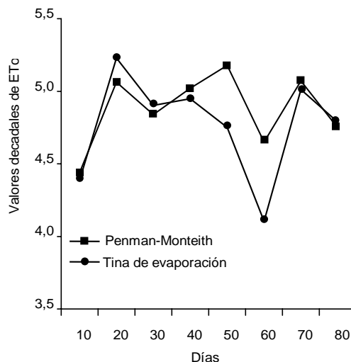
Figura 3. Valores decadales de ET_0 usando los métodos de la tina de evaporación y Penman-Monteith durante el período 1 (abril-julio 2001).
