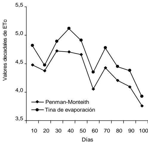
Figura 4. Valores decadales de ET_0 usando los métodos de la tina de evaporación y Penman-Monteith durante el período 2 (julio-noviembre 2001).
