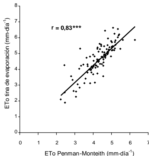
Figura 2. Valores diarios de ET_0 usando los métodos de Penman-Monteith y tina de evaporación en el período 2 (julio-noviembre 2001)
