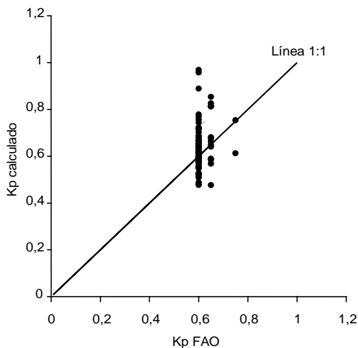
Figura 5. Relación entre el K_p tabulado y el K_p calculado durante el período 1 (abril-julio 2001).
